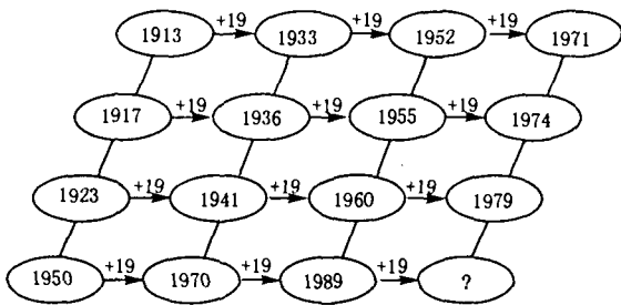
图 2 20 世纪以来川滇地区发生 \geq 6.7 级地震的部分年份关系图
